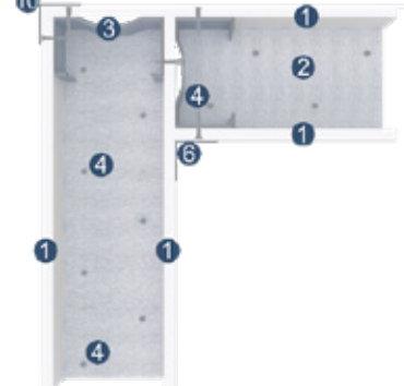
* Detalle 3: Encuentro en L
